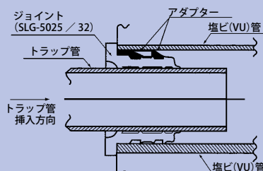
《SLG-4025/32・SLG-5025/32 取付詳細図》
